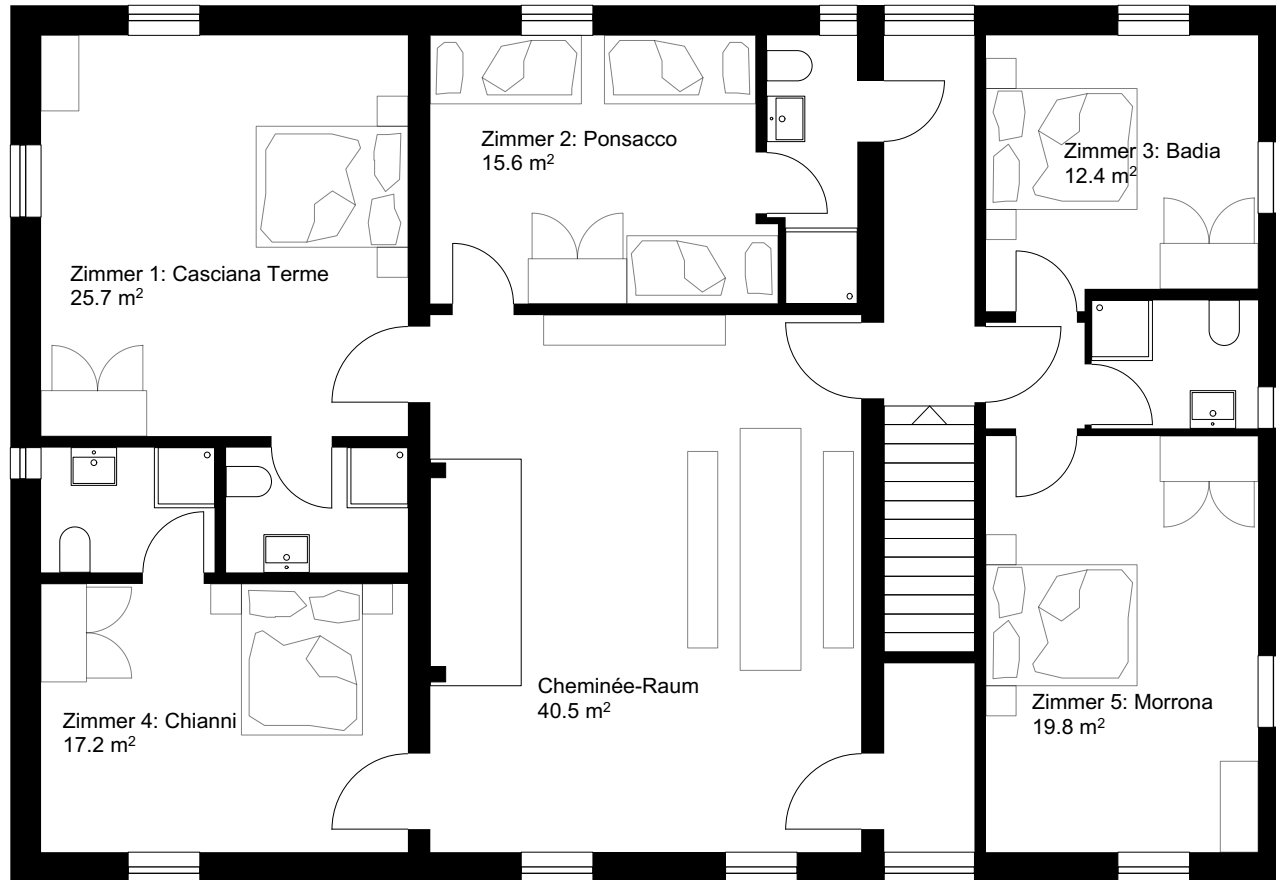
Obergeschoss
